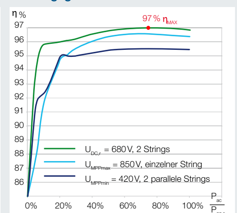
Wirkungsgradkennlinien PIKO 10.1
