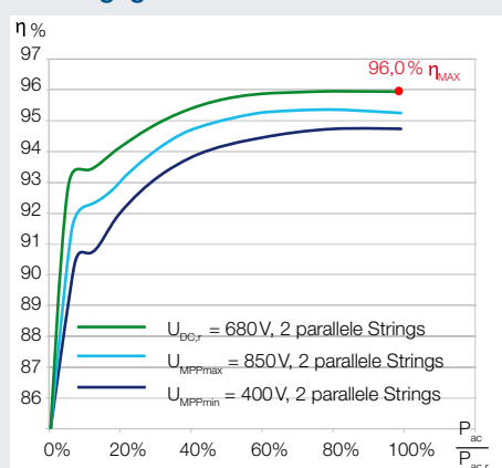
Wirkungsgradkennlinien PIKO 7.0
